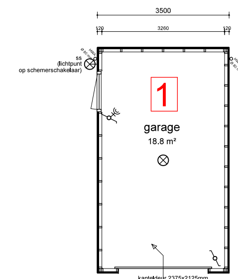
BEGANEGROND (optie 1)
