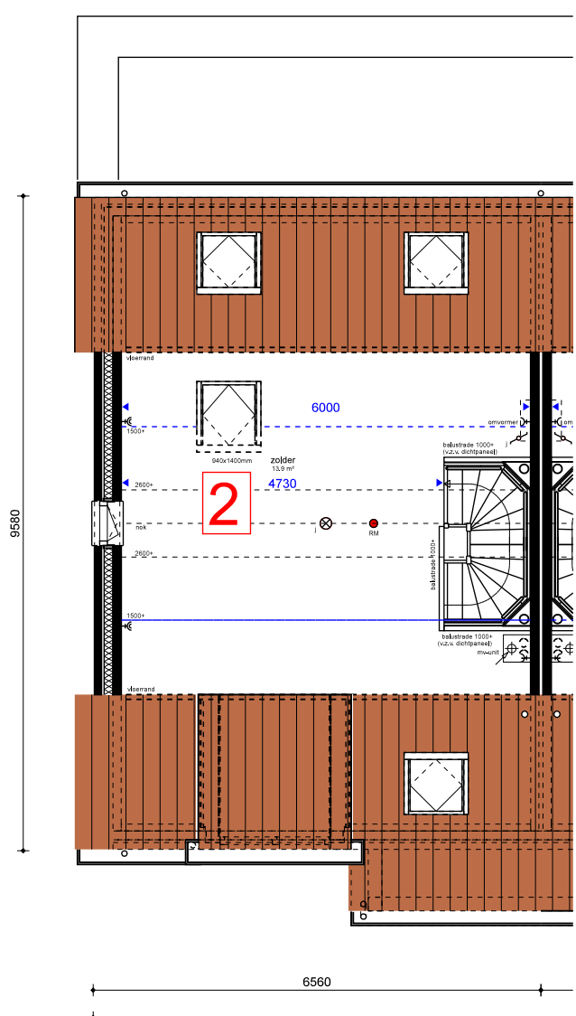
ZOLDER (optie 2)
