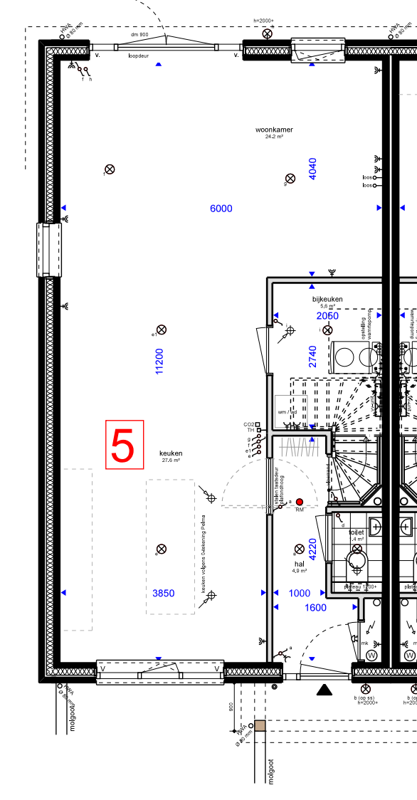
BEGANEGROND (optie 5)
