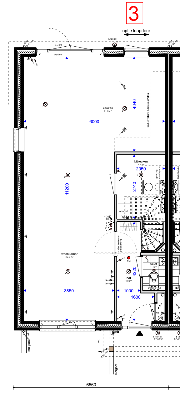
BEGANEGROND (optie 3)
